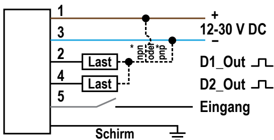
Abbildung 9. Ausführungen mit doppeltem Schaltausgang
