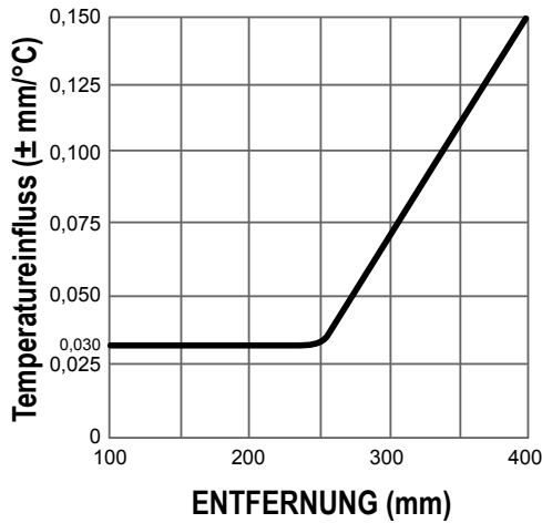
Abbildung 16. Temperatureinfluss
