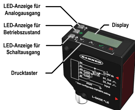
Abbildung 1. Funktionen des LE-Sensors mit doppeltem Schaltausgang
