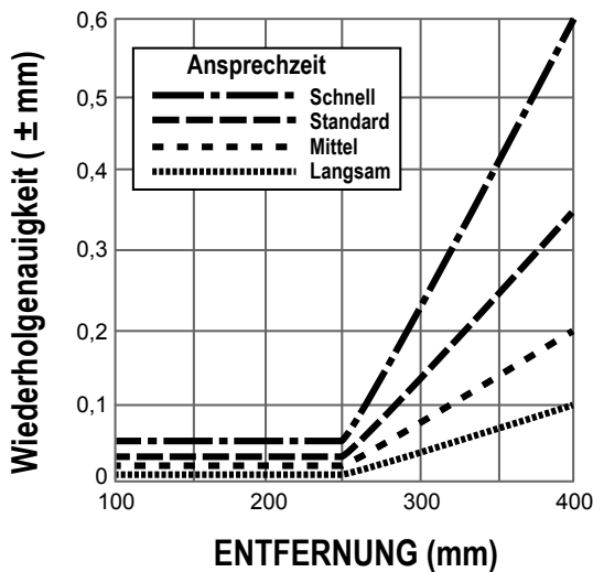
Abbildung 14. Wiederholgenauigkeit (90 % bis 6 % Reflexionsvermögen)
