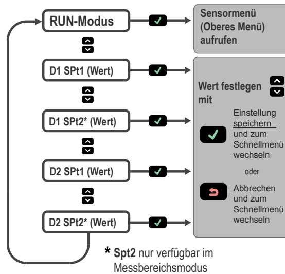
Abbildung 12. Übersicht über das Schnellmenü (Betriebsart "Fenster")
