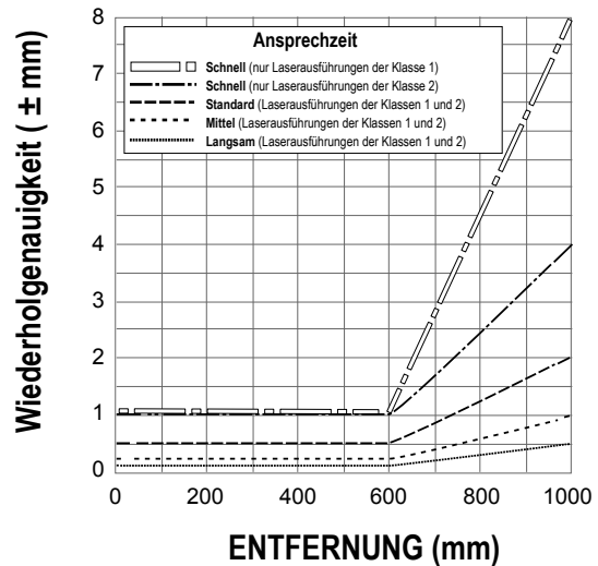
Abbildung 15. Wiederholgenauigkeit (90 % bis 6 % Reflexionsvermögen)
