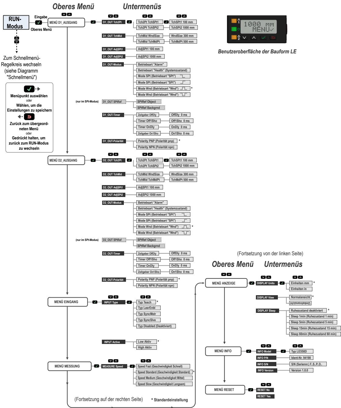
Abbildung 13. LE550-Sensormenü – Übersicht (Ausführungen mit doppeltem Schaltausgang)
