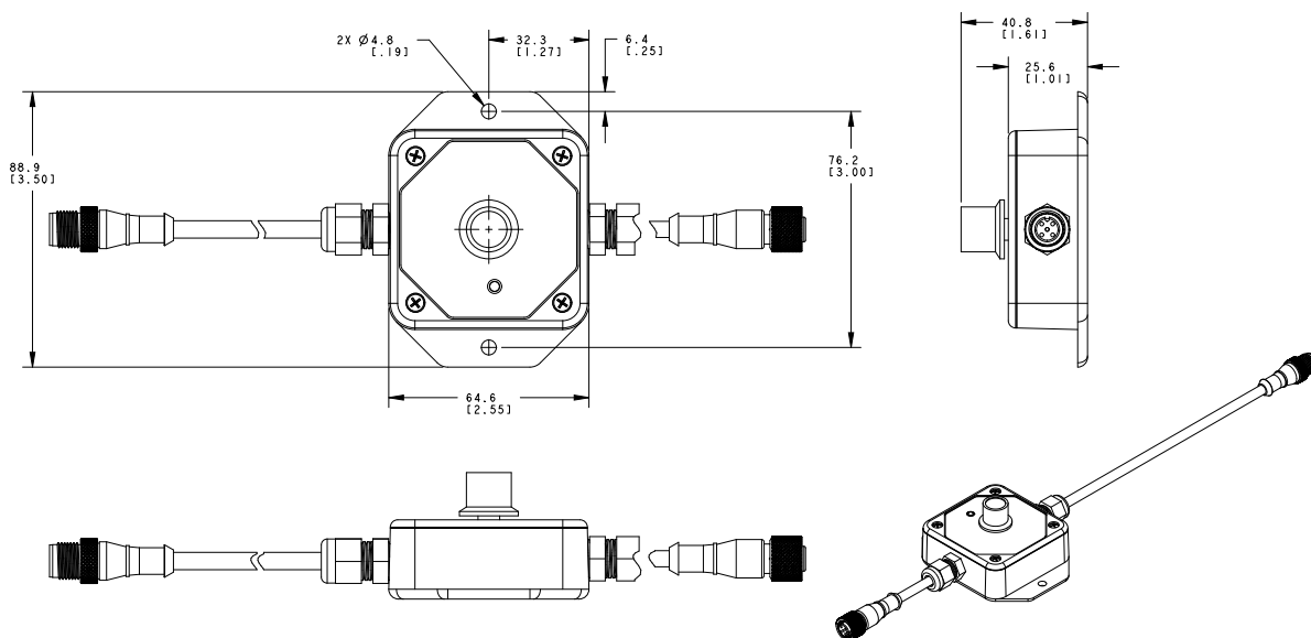
Abbildung 2. Kabelgebundene Modelle
