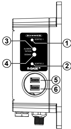
Illustration 1. Caractéristiques R-GAGE
