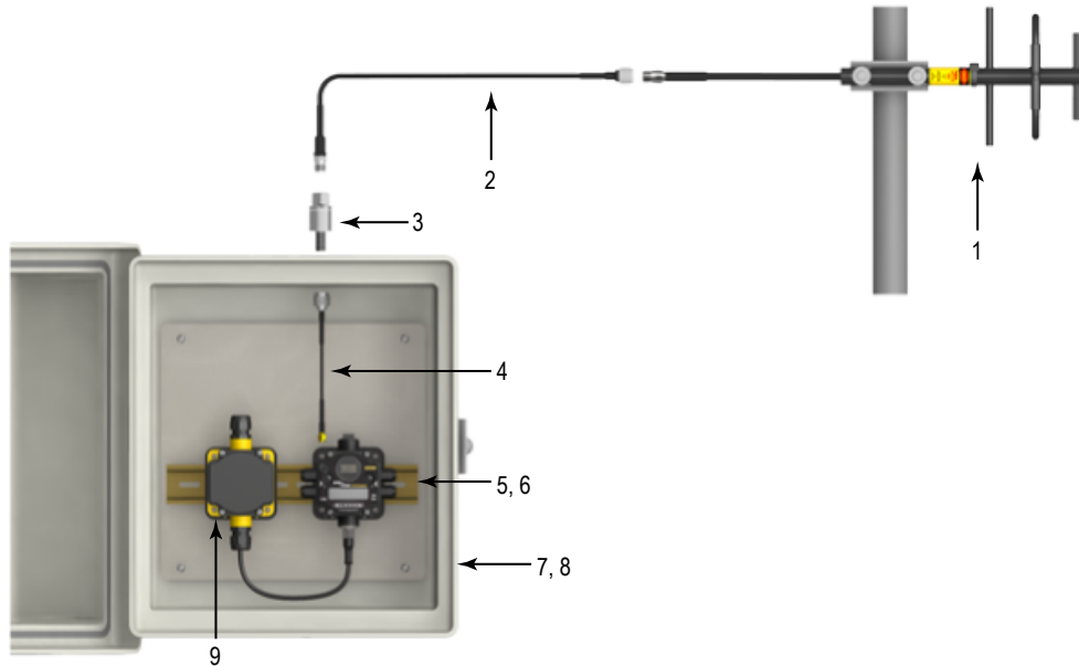
Composants nécessaires au montage d'une antenne sur un poteau
