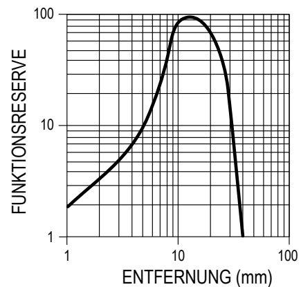
Funktionsreservekurve mit 40 mm Ausblendgrenze (bei weißer Karte mit 90% Reflexionsvermögen)
