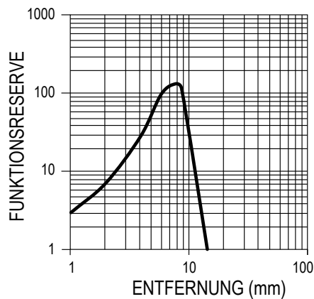
Funktionsreservekurve mit 15 mm Ausblendgrenze (bei weißer Karte mit 90% Reflexionsvermögen)
