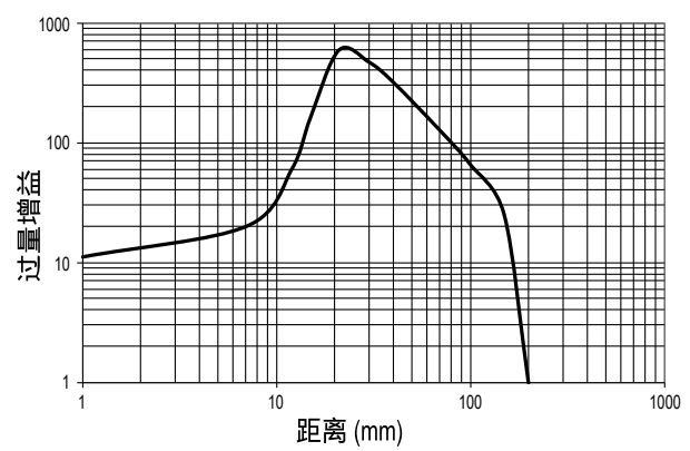
截止距离为 200 毫米的过量增益曲线 (基于 90% 白卡)
