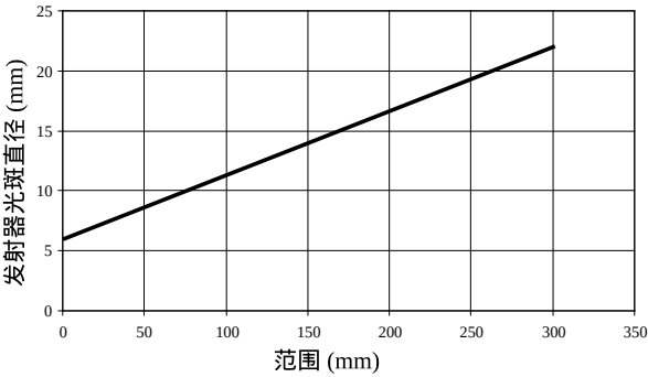
典型发射器光斑直径与距离的关系
