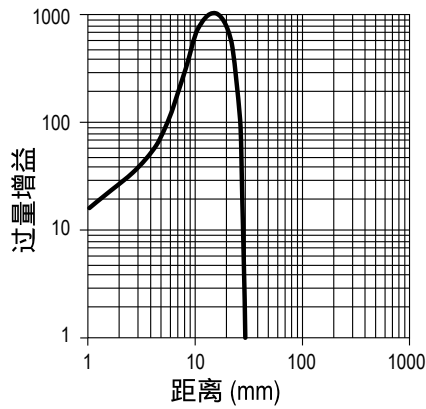
截止距离为 30 毫米的过量增益曲线 (基于 90% 白卡)
