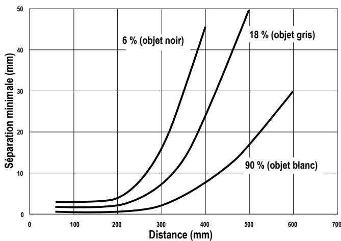
Illustration 7. Distance de séparation* minimale entre l'objet et l'arrière-plan : mode à suppression d'arrière-plan
