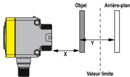
Illustration 7. Distance de séparation* minimale entre l'objet et l'arrière-plan : mode à suppression d'arrière-plan
