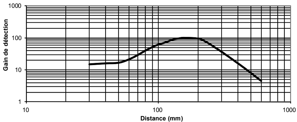
Illustration 8. Courbes de réserve de gain du QS30AF600 (sur la base d'une carte blanche 90 %)
