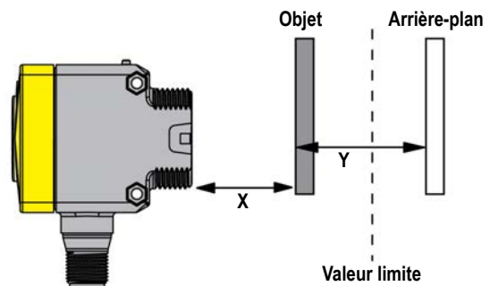
Illustration 3. Régler la distance limite environ à mi-chemin entre la cible la plus éloignée et l'arrière-plan le plus proche
