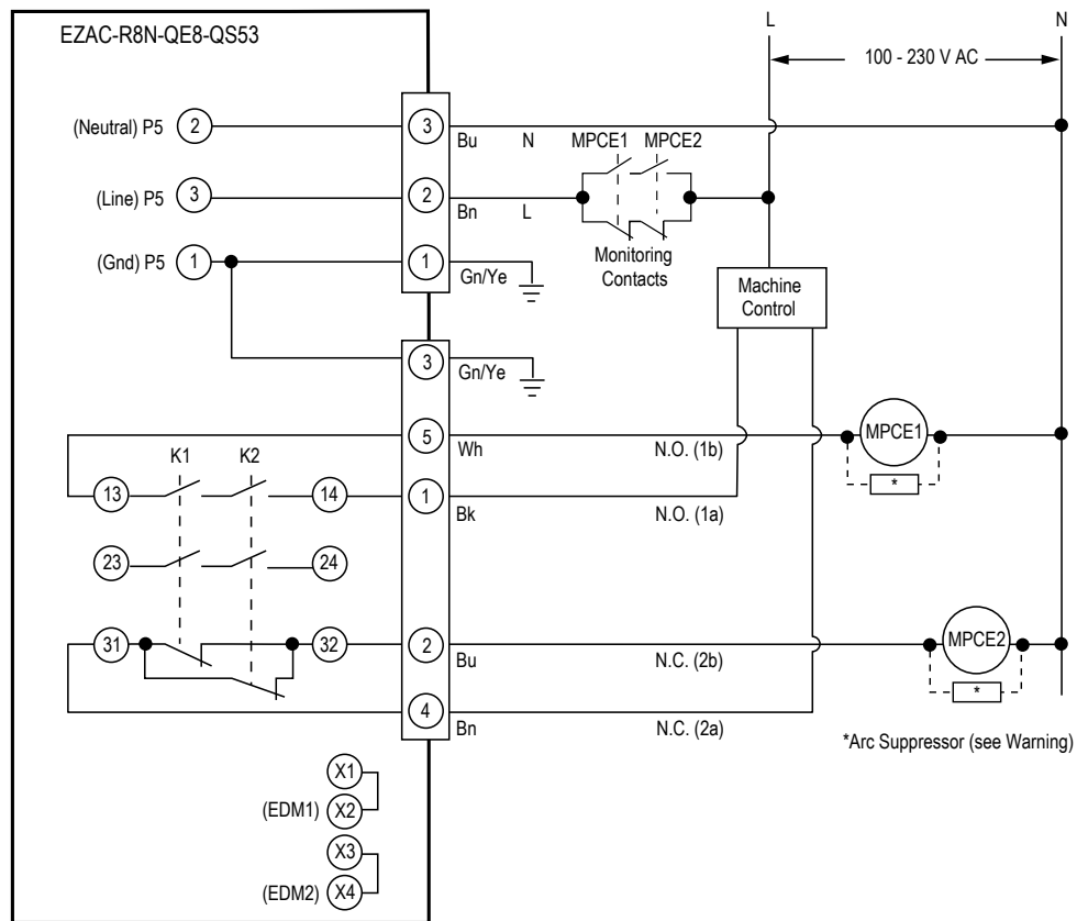
Wiring—model EZAC-R8N-QE8-QS53
