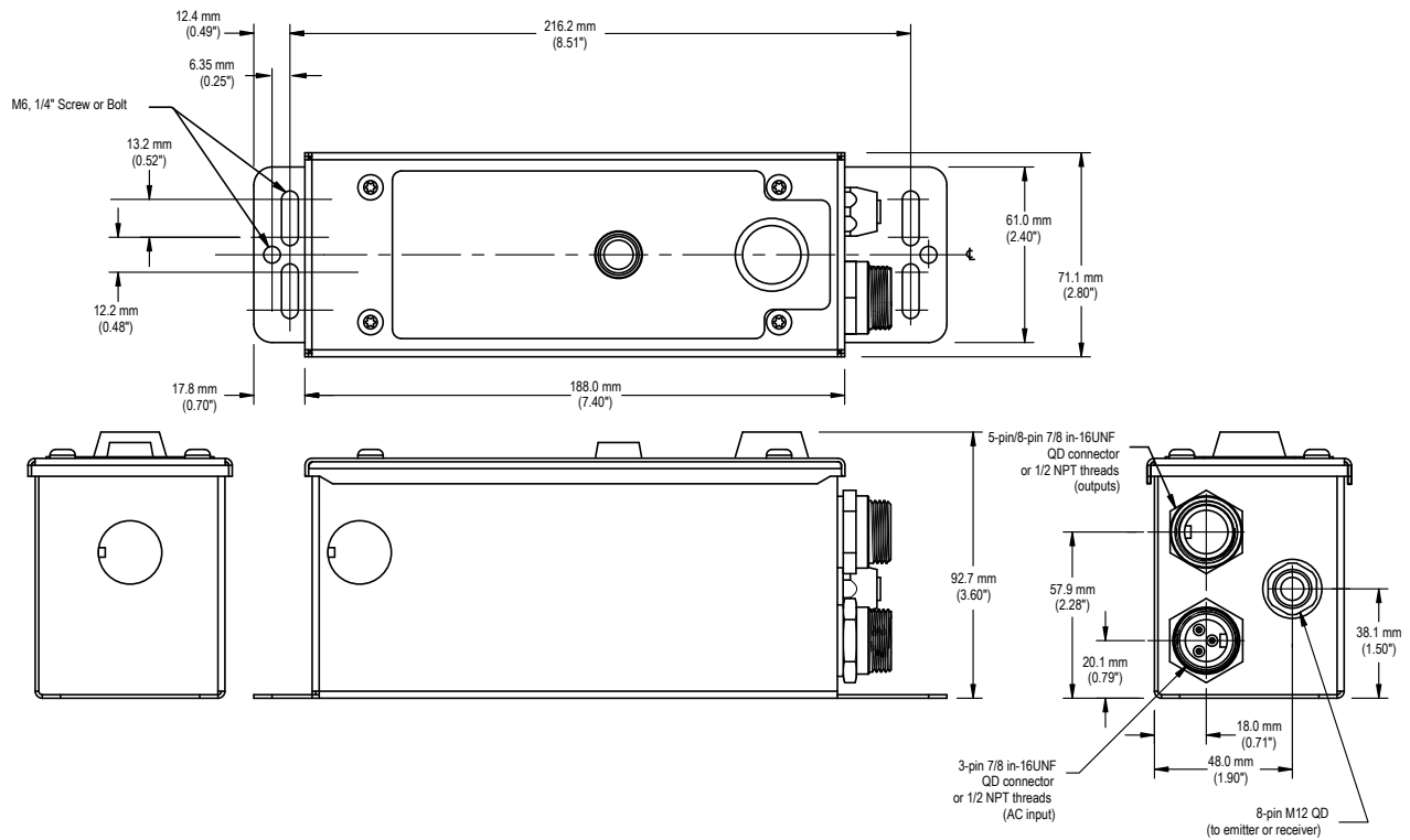
Model EZAC-R.. EZ-SCREEN AC Interface Box
