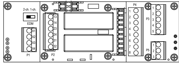
Wiring—model EZAC-R11-QE8
