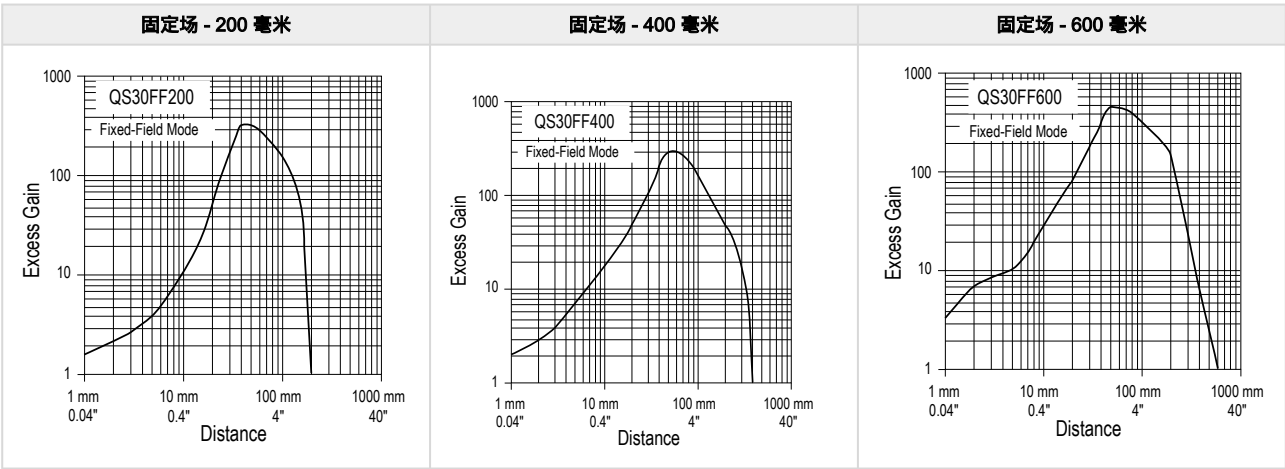
固定场式传感器过量增益 (3)
