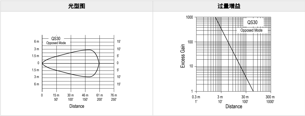
偏光反射板式传感器 (2)
