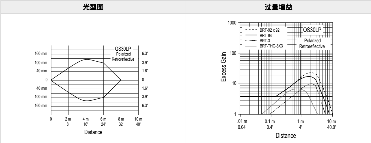
固定场式传感器过量增益 (3)
