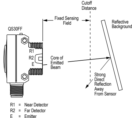
超出截止距离的目标 - 解决方法
