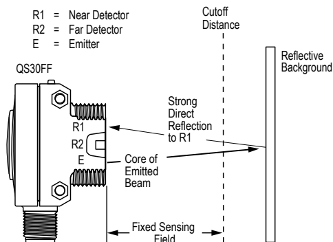
超出截止距离的目标 - 问题
