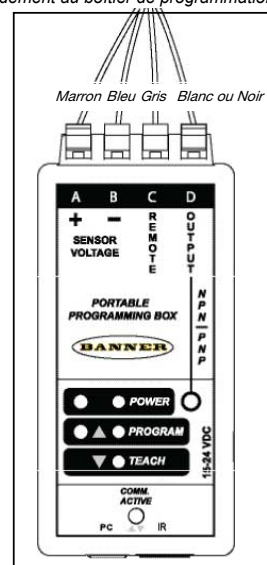
Illustration 7. Raccordement au boîtier de programmation portable modèle DPB1
