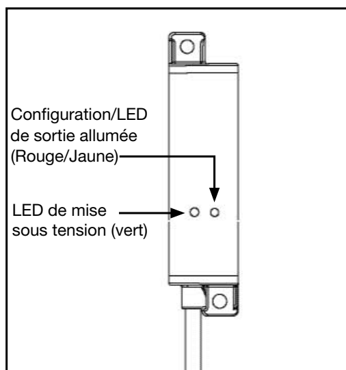
Illustration 6. Caractéristiques du capteur
