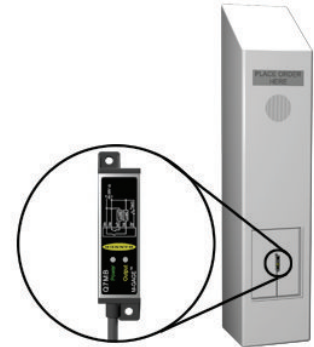
Illustration 3. Installation à l'aide des trous de montage dans les embouts du capteur
