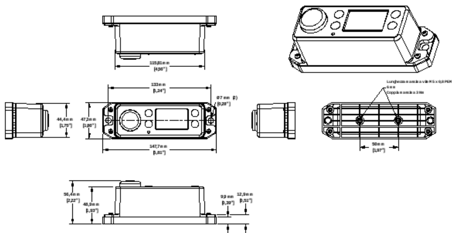
Figura 4. Dimensioni DSTS CB
