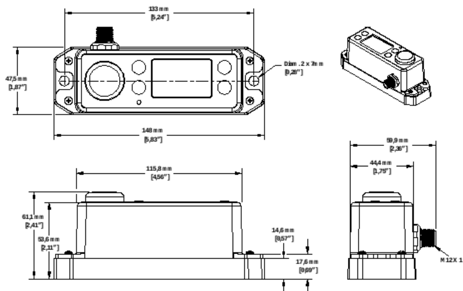
Figura 4. Dimensioni DSTS CB
