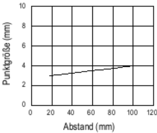
Q2XLAF100 (Laser) – Typischer Sender-Punktdurchmesser im Vergleich zum Abstand
