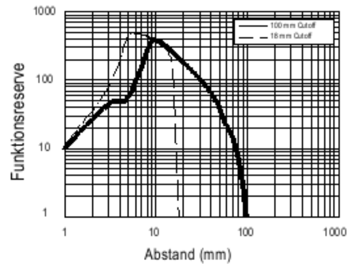
Q2XLAF100 (Laser) – Funktionsreservekurve mit Ausblendgrenzen bei 18 mm und bei 100 mm (basierend auf 90 % weiße Karte)
