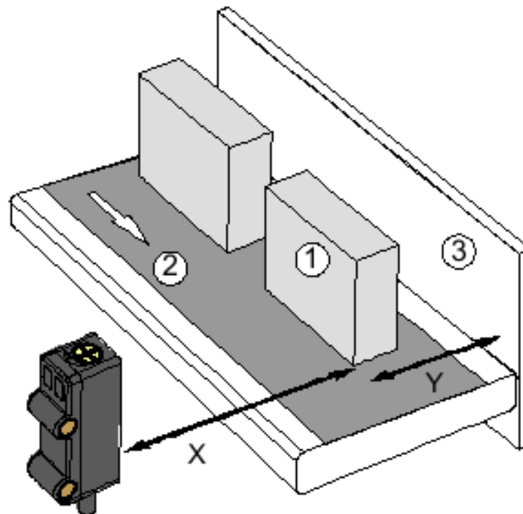
Anwendungsbeispiel für Modus „Hintergrundaussblendung“
