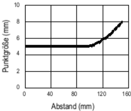
Q2XAF150 (LED) – Typischer Sender-Punktdurchmesser im Vergleich zum Abstand
