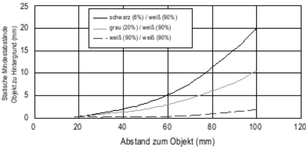
Q2XLAF100 (Laser) – Statischer Mindestsicherheitsabstand zwischen Objekt und Hintergrund: Modus „Hintergrundaussblendung“
