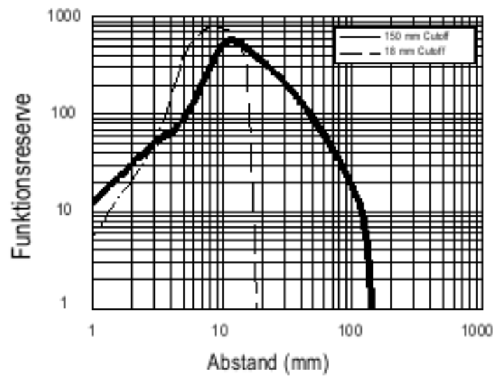
Q2XAF150 (LED) – Funktionsreservekurve mit Ausblendgrenzen bei 18 mm und bei 150 mm (basierend auf 90 % weiße Karte)
