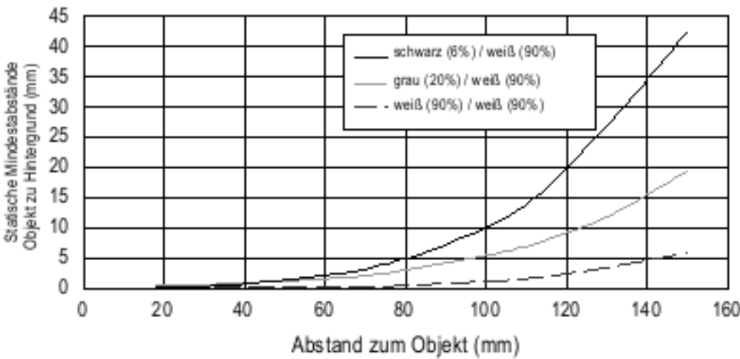
Q2XAF150 (LED) – Statischer Mindestsicherheitsabstand zwischen Objekt und Hintergrund: Modus „Hintergrundaussblendung“
