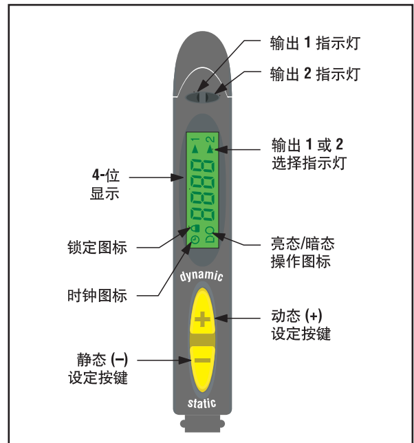
图1. D10 指示灯
