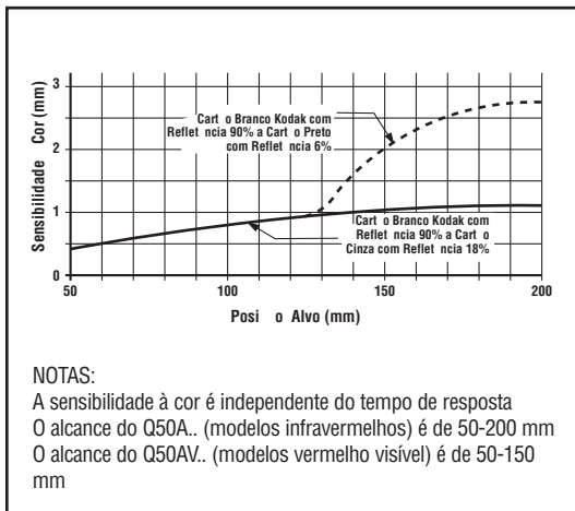
Figura 4. Sensibilidade à Cor do Sensor L-GAGE Q50A com Saídas Digitais e Complementares versus Posição (Isto representa a mudança esperada na saída quando a cor do alvo é mudada de um Cartão Branco Kodak com reflexo de 90% para uma superfície com reflexo de 6% e 18%.)
