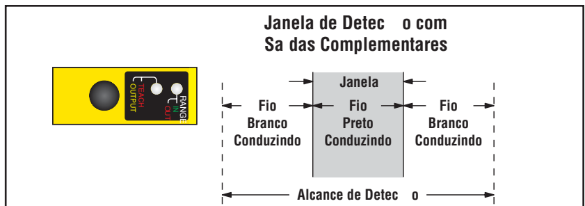
Figura 5. Programando um par simples de limites de janela de detecção, saídas complementares
