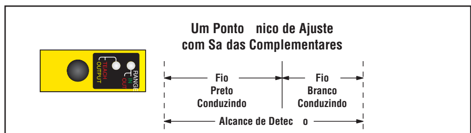
Figura 7. Programando limites de ponto de ajuste de detecção separados, saídas complementares
