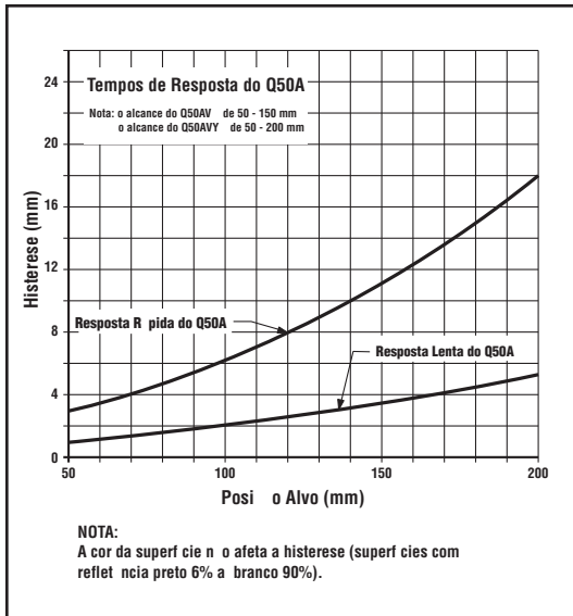
Figura 3. Histerese vs. Posição do L-GAGE Q50A (Digital e Complementar)
