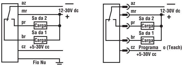
Esquema de Ligação NPN Modelos com Cabo Modelos com Desconexão Rápida
