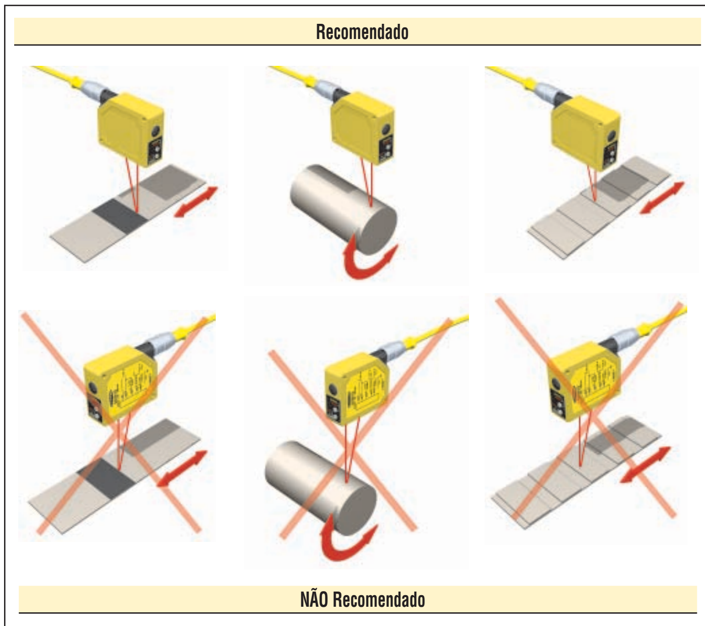
Figura 8. Orientações de sensores para alvos típicos
