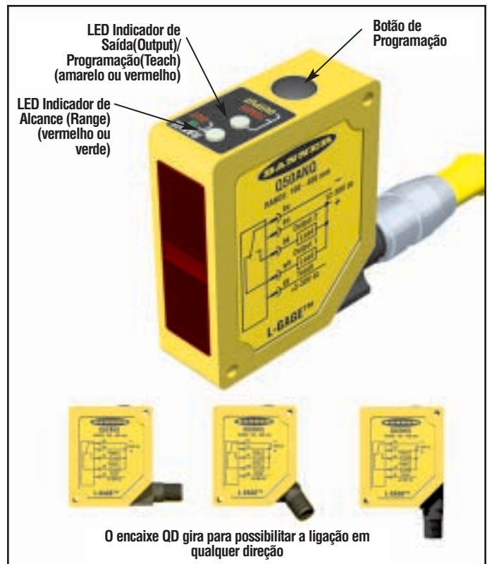
Figura 2. Características do sensor L-GAGE Q50A
