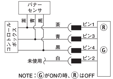
2カラー(..RGX7P..) モデル
