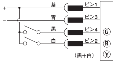
PNP(..GXRP..) 3色モデル
