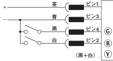
NPN(..GXRN..) 3色モデル
