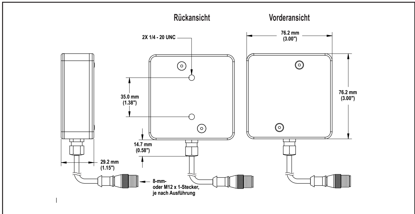
Abbildung 1. Abmessungen der Flächenbeleuchtung
