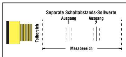
Abbildung 2b. Programmierung separater Schaltabstands-Sollwerte
