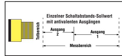
Abbildung 2d. Programmierung separater Schaltabstands-Sollwerte, antivalente Ausgänge
