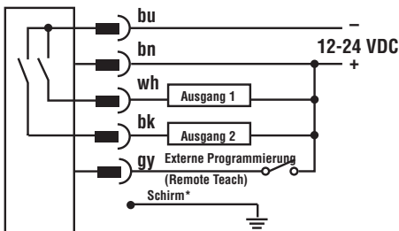
npn-Steckergeräte
