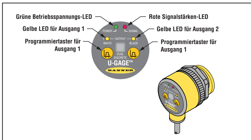
Abbildung 1. Programmier- und Anzeigen des U-GAGE -Sensors Bauform T30
