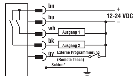
pnp-Steckergeräte
