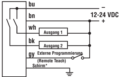
npn-Steckergeräte
