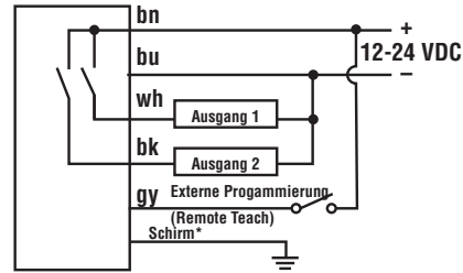
pnp-Steckergeräte
