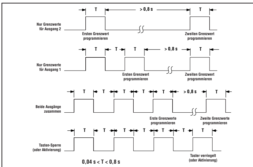
Abbildung 3. Zeitablaufprogramme für externe Programmierung (Remote TEACH-Prozeduren)
