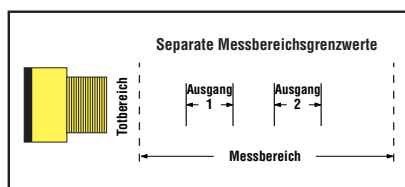
Abbildung 2a. Programmierung separater Messbereichsgrenzwerte
