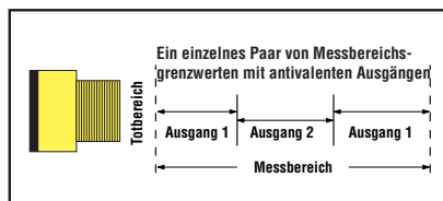
Abbildung 2c. Programmierung eines einzelnen Paares von Messbereichsgrenzwerten, antivalente Ausgänge
