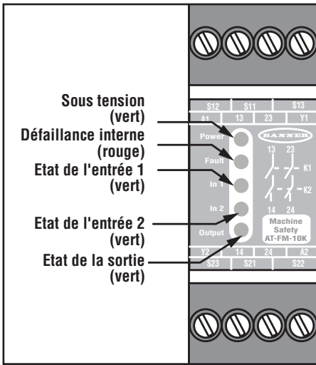
Figure 1. Voyants d'état AT-FM-10K
