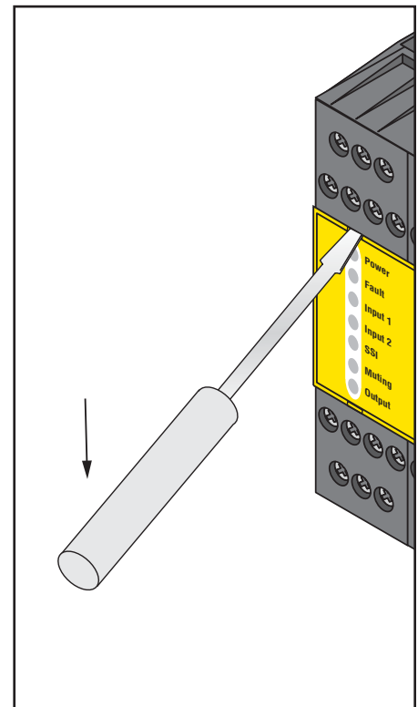
Figure 6. Pour retirer un bornier, insérer un petit tournevis dans la fente indiquée et faire levier pour le détacher.
