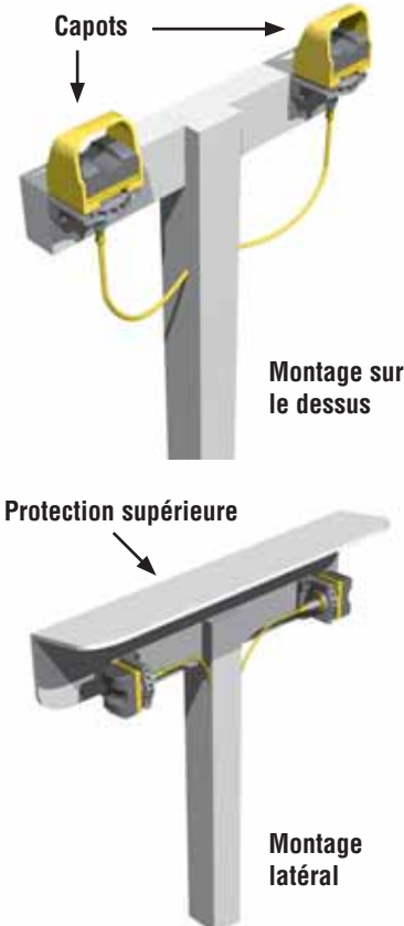
Figure 3. Installer les dispositifs d'activation pour qu'ils soient protégés contre une utilisation frauduleuse ou accidentelle (l'illustration représente des boutons tactiles Banner STB)
