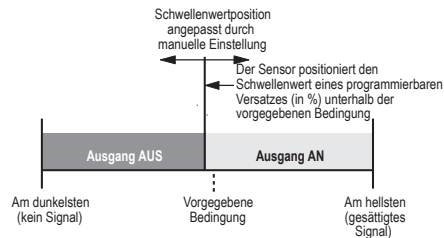
Abbildung 5. Hell-Einstellung (Hellschaltung dargestellt)
