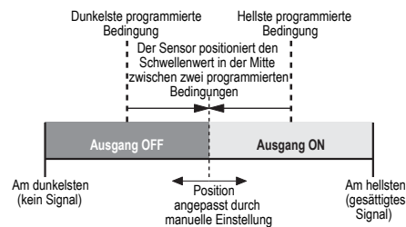
Abbildung 2. Zweipunkt-TEACH-Programmierung (Hellschaltung dargestellt)
