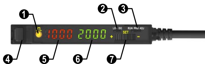
Figura 1. DF-G1 - Caratteristiche del modello
