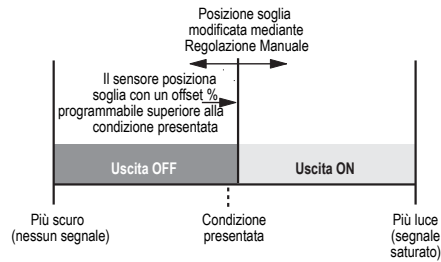
Figura 6. Dark SET (in figura, modalità luce)
