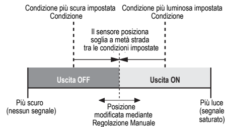
Figura 2. TEACH con impostazione di due posizioni (in figura, modalità luce)
