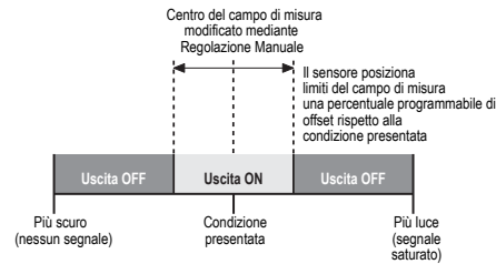
Figura 4. Window SET (in figura, modalità luce)
