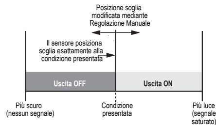
Figura 7. Calibration SET (in figura, modalità luce)
