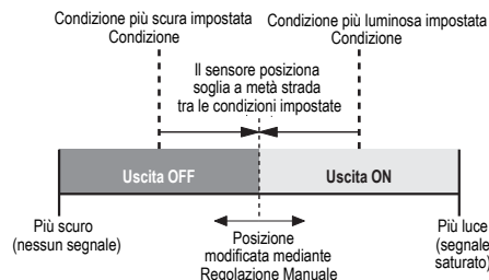
Figura 3. Dynamic TEACH (in figura, modalità luce)
