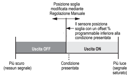
Figura 5. SET Luce (in figura, modalità luce)
